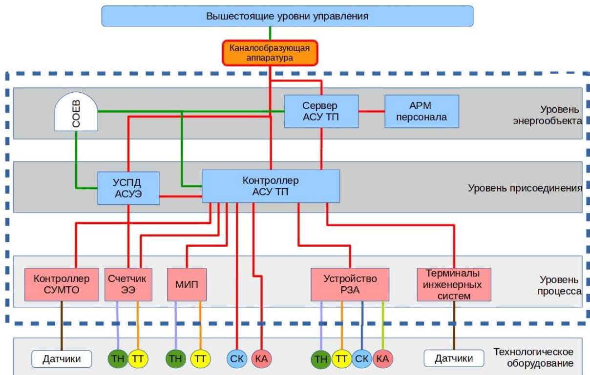
Рисунок 3. Централизованная архитектура
